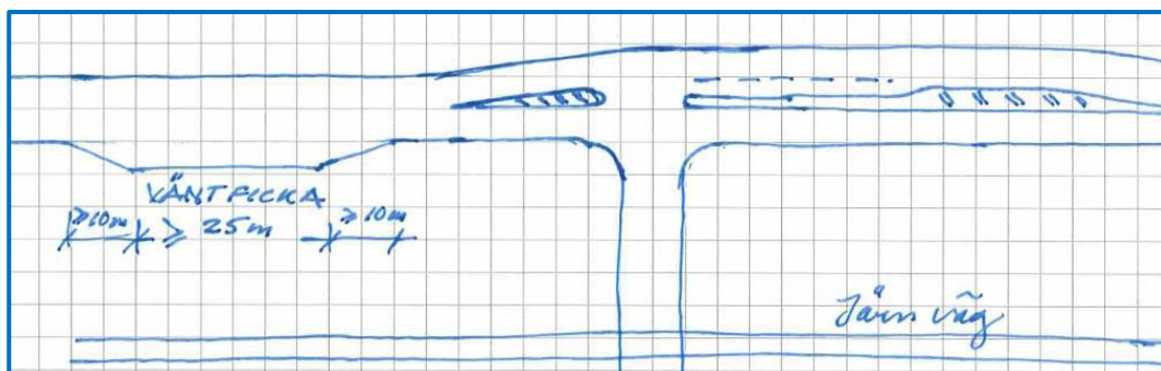
Bild 25. Väntficka för högersvängande och vänstersvängfält.
